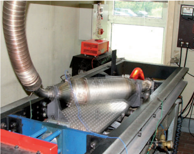
Unser Hot-Shake-Prüfstand simuliert in geraffter Form die mechanischen Belastungen unter den zyklischen Abgastemperaturen, die ein Autoleben mit sich bringt.
